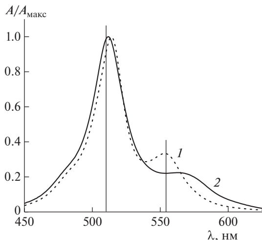
Рис. 4. Нормированные спектры поглощения бис-ТКЦ ( 2.7 \times 10^{-6} моль л ^{-1} ) в воде в присутствии КБ7 ( 1 \times 10^{-3} моль л ^{-1} ) (спектр 1) и КБ8 ( 5 \times 10^{-3} моль л ^{-1} ) (спектр 2). Вертикальными линиями отмечены максимумы поглощения бис-ТКЦ в отсутствие кавитандов.
